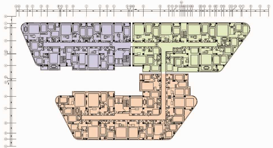
پلان کلی جانمایی بلوک های سه گانه A, B, C برج مسکونی نارنجستان چهار
