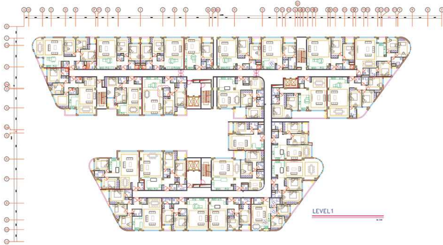
پلان کلی جانمایی واحدهای طبقه یک، بلوک های سه گانه A, B, C برج مسکونی نارنجستان چهار
