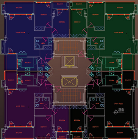
پلان طبقات اول تا پنجم ، هر واحد ۱۱۸ متر مربع
