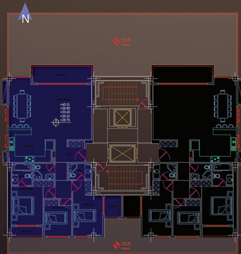
پلان طبقات ششم تا یازدهم ، هر واحد ۱۵۵ متر مربع
